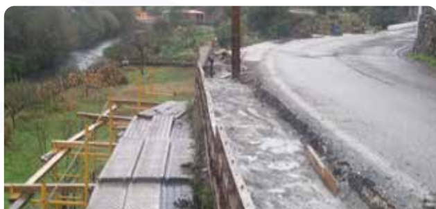
Construção de muro de suporte para posterior colocação de guardas metálicas na Estrada do Pombal – Pampilhosa da Serra
